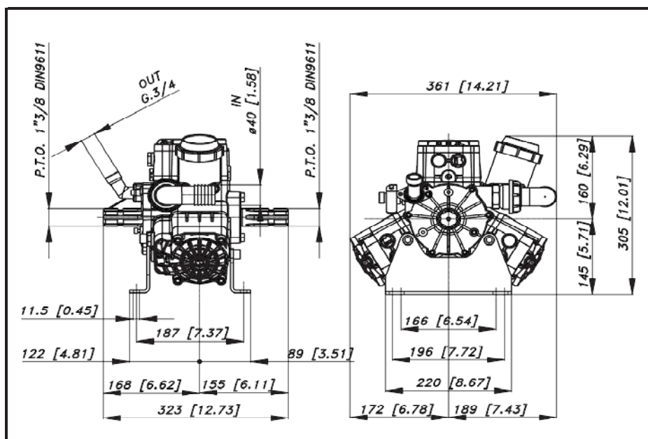
ALBERO POMPA VD - VD PUMP SHAFT
