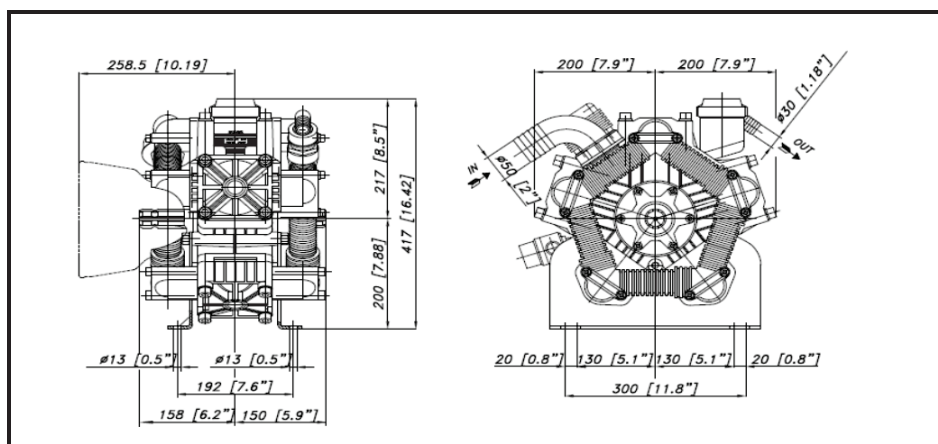
DIMENSIONI D'INGOMBRO - OVERALL DIMENSIONS
